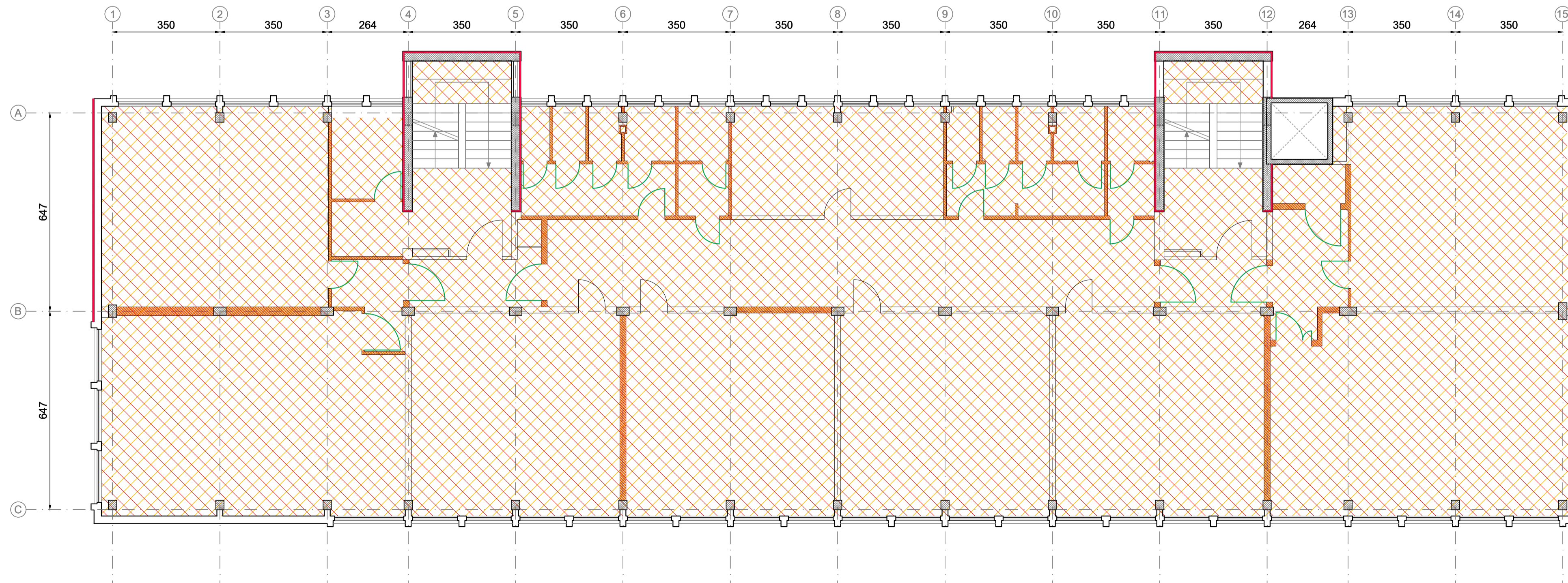
PIANO PRIMO scala 1:100
