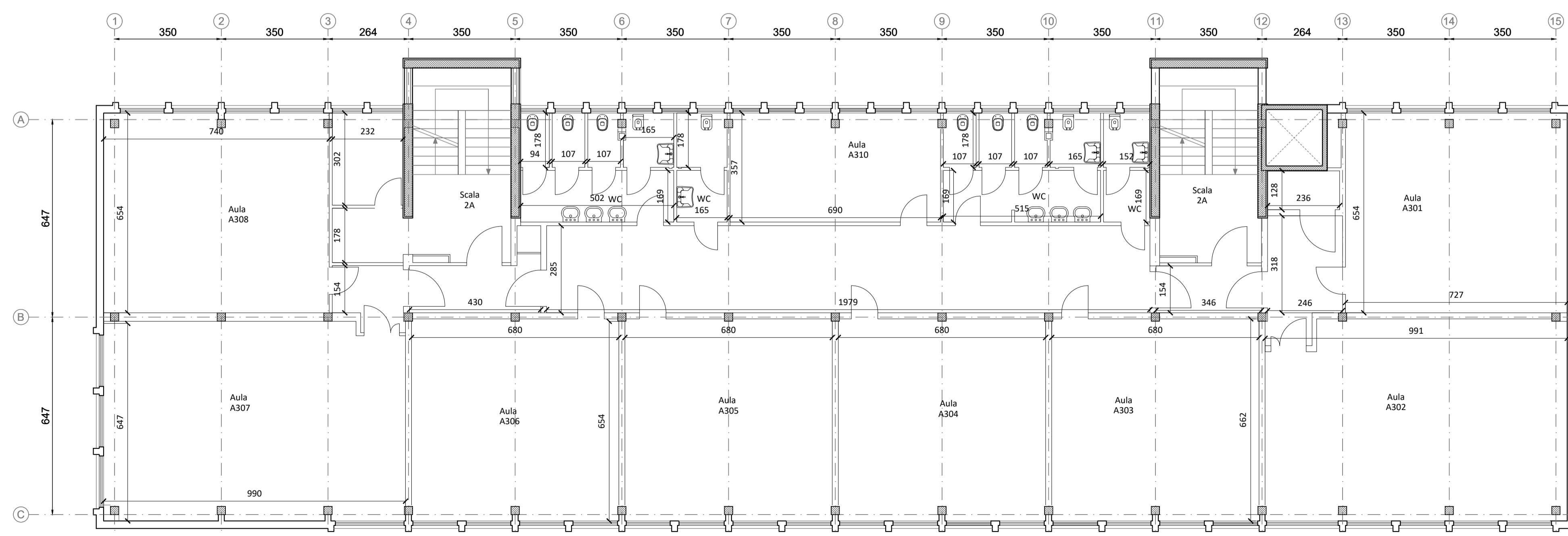
PIANO TERZO scala 1:100
