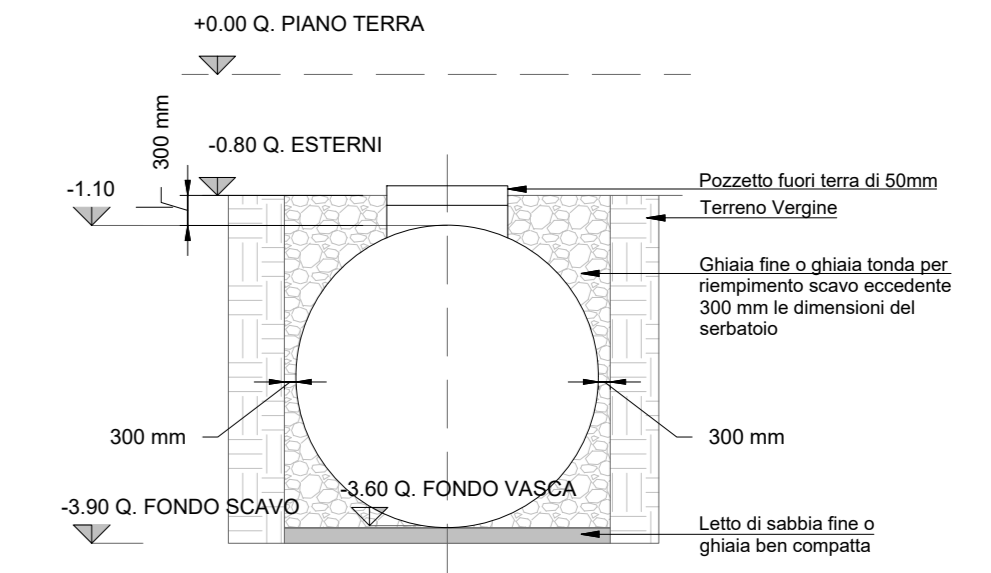
CISTERNA CILINDRICA DA INTERRO De 250 x 490 cm SEZIONE LONGITUDINALE
