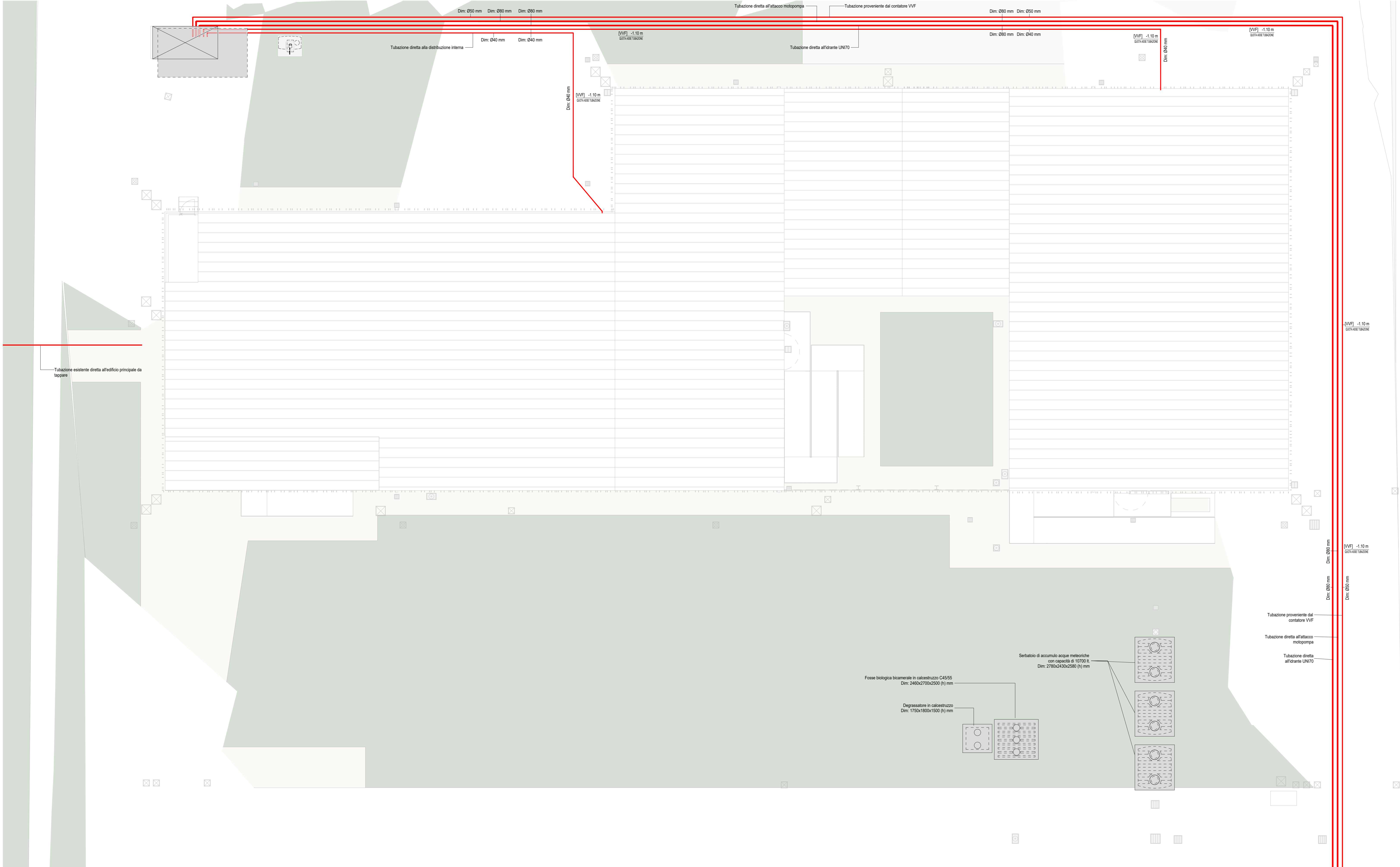
P0 - Impianto antincendio - Esterno Scala 1 : 100
