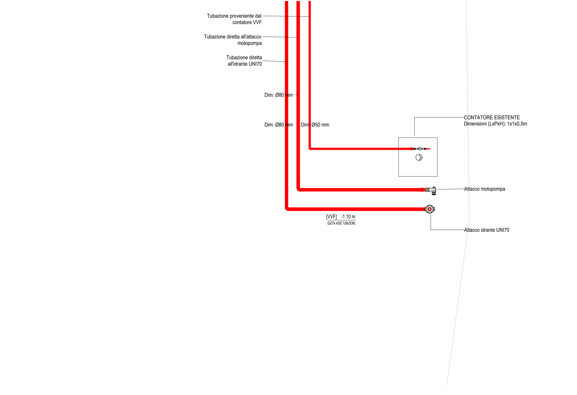
Particolare A - Zona contatore Scala 1 : 50
