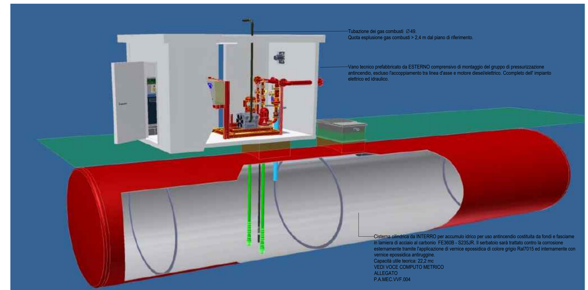
A-P --- Locale antincendio
