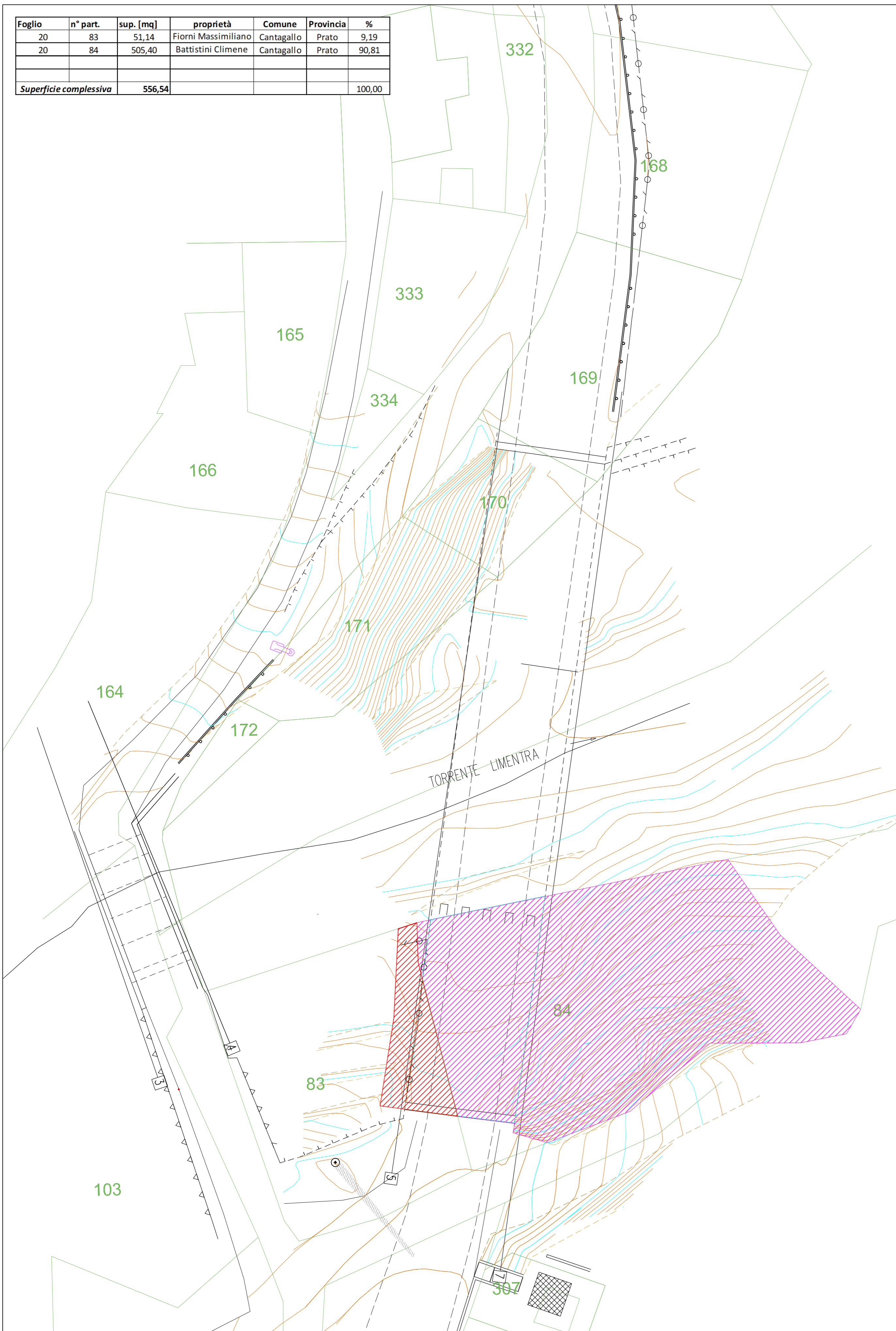
Piano particellare: occupazioni temporanee - scala 1:200
