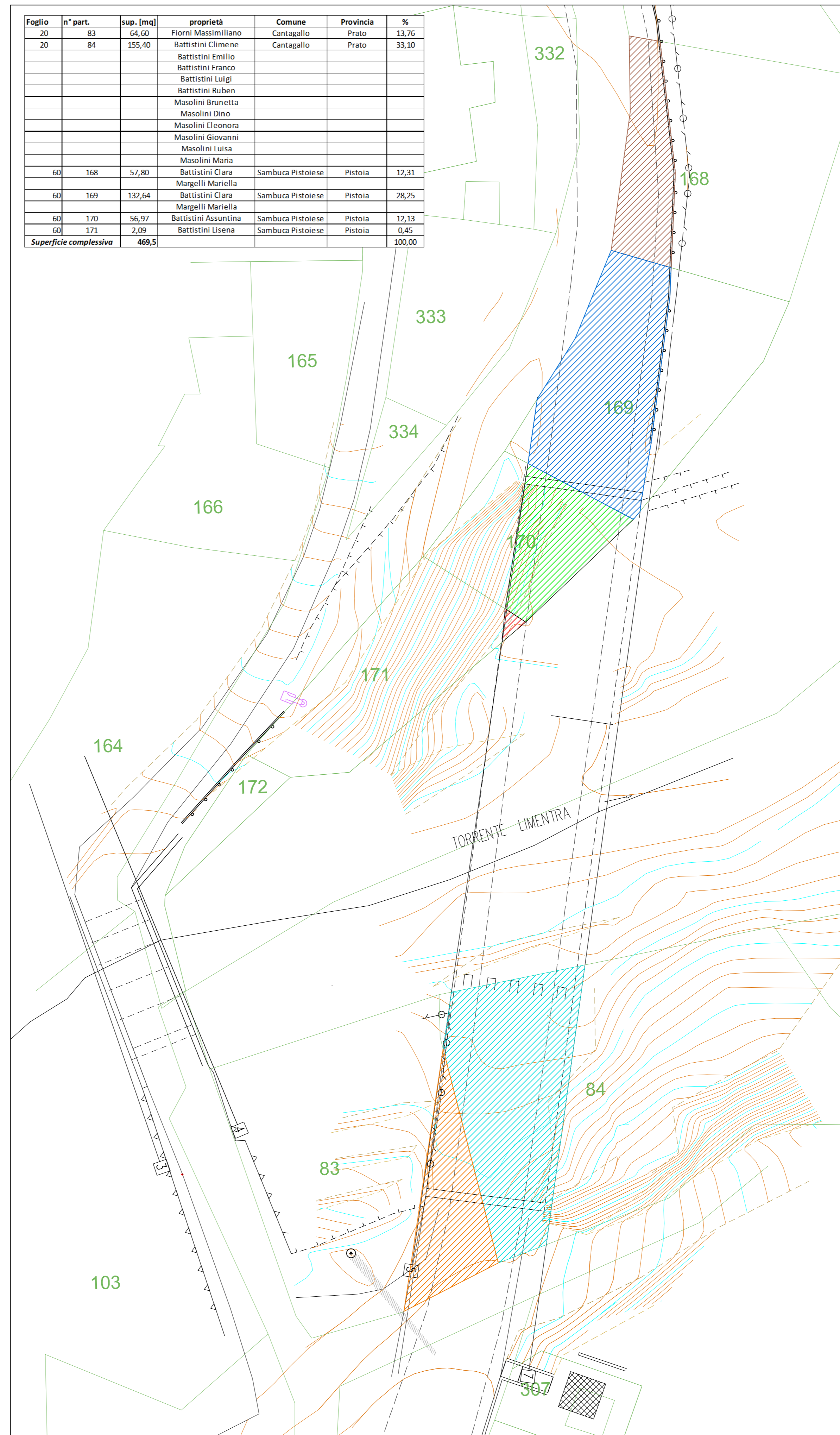
Piano particellare: aree interessate dall'infrastruttura ponte e viabilità - scala 1:200
