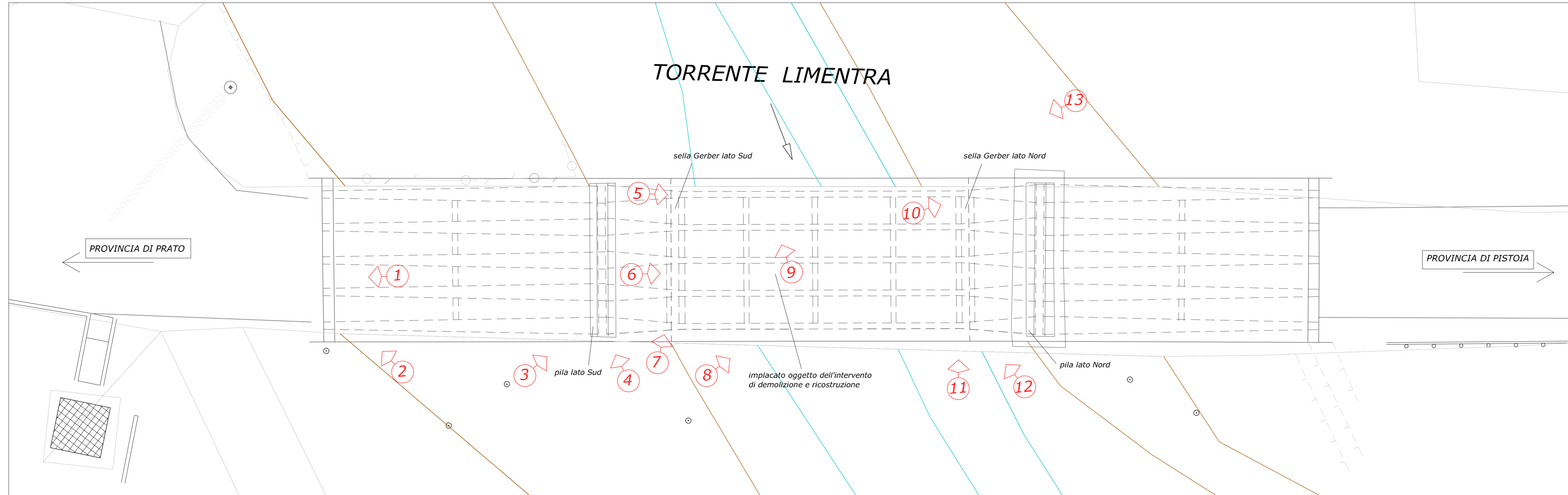
Planimetria generale - scala 1:100
